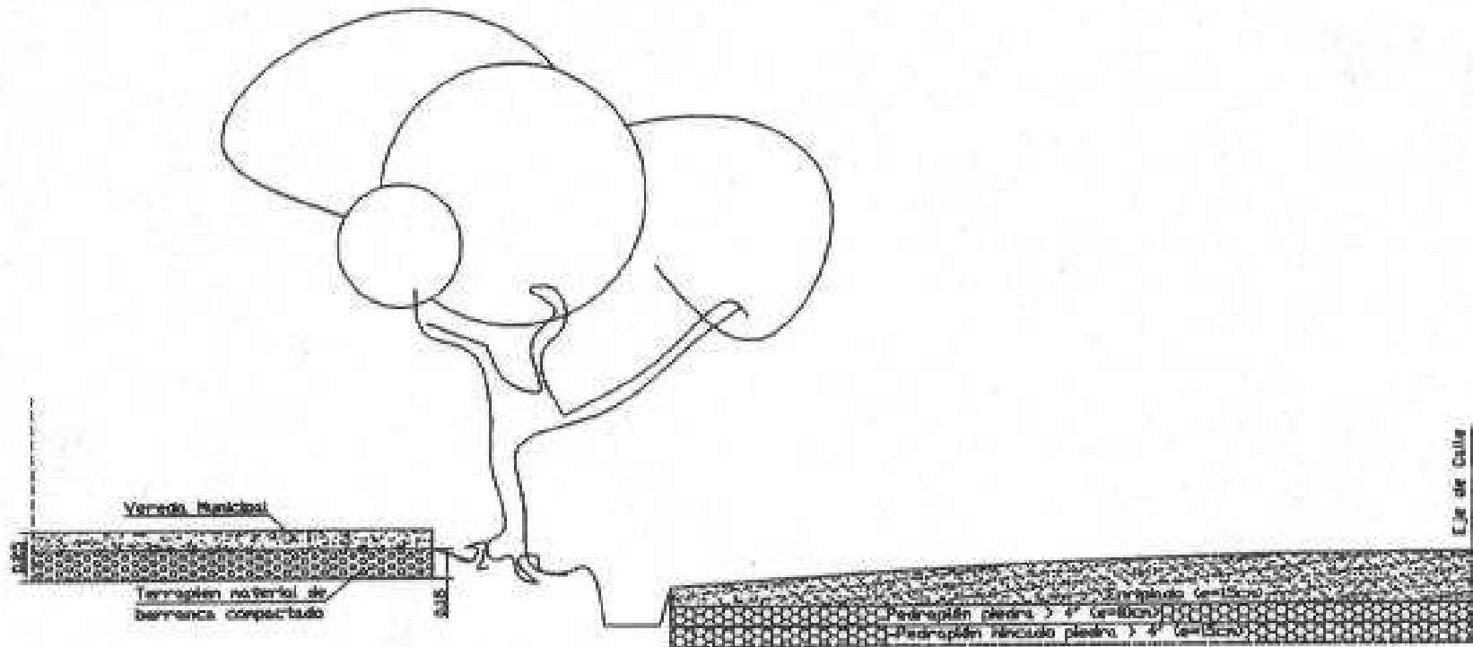
DETALLE DE MEJORAMIENTO DEL TERRENO BAJO VEREDAS Y CALLES
